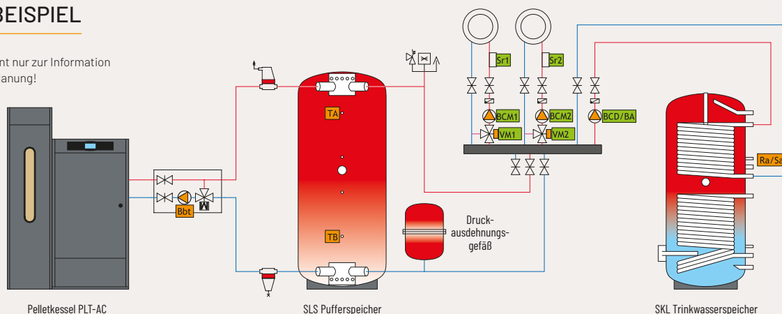
Pelletkessel PLT-AC
